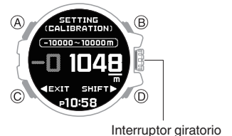
Interruptor giratorio
