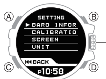
Interruptor giratorio
