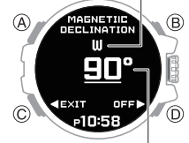
Ángulo de la declinación magnética
